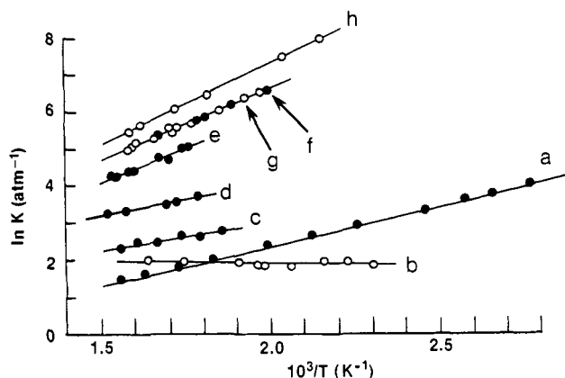
Figure 6. van't Hoff plots for proton-transfer equilibria between the reactants: a. azuleneH + + N,N -dimethylaniline; b. i -C 3 H 7 NH 3 + + azulene; c. CH 3 OCH 3 H + + i -C 4 H 8 ; d. CH 2 CHCNH + + CH 3 OCH 3 ; e. i -C 4 H 9 + + CH 3 SCH 3 ; f. i -C 4 H 9 + + CH 3 COOC 2 H 5 ; and g. i -C 4 H 9 + + (C 2 H 5 ) 2 CO.
