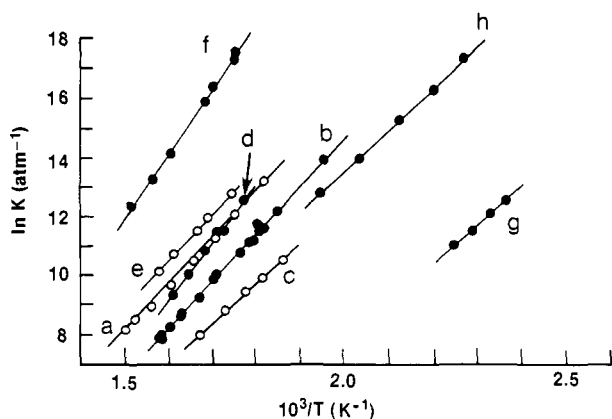
Figure 12. van't Hoff plots for equilibria for association reactions between the reactants: a. (\text{CH}_3)_2\text{OH}^+ + (\text{CH}_3)_2\text{O} ; b. t\text{-C}_3\text{H}_7^+ + \text{H}_2\text{S} ; c. \text{NH}_4^+ + \text{NH}_3 ; d. t\text{-C}_3\text{H}_7^+ + \text{HCN} ; e. (\text{CH}_3)_2\text{COH}^+ + (\text{CH}_3)_2\text{CO} ; f. t\text{-C}_4\text{H}_9^+ + (\text{CH}_3)_2\text{S} ; g. t\text{-C}_3\text{H}_7^+ + \text{H}_2\text{O} ; and h. \text{C}_6\text{H}_5\text{COCH}_2\text{H}^+ + \text{C}_6\text{H}_5\text{COCH}_3 .
